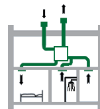
Řízené větrání obytného prostoru
